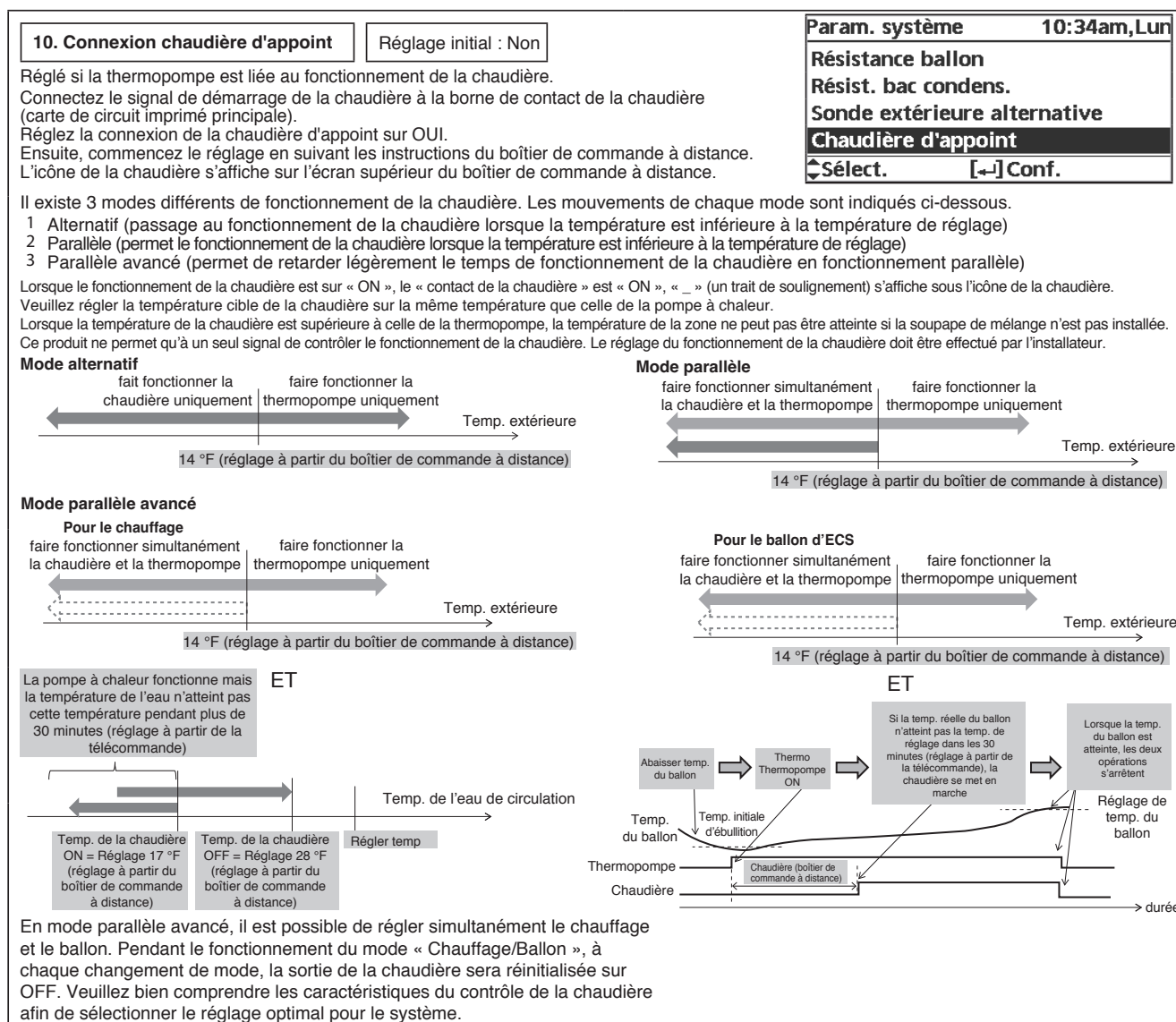
Figure 6-26 Paramètres du boîtier de commande à distance (suite)
