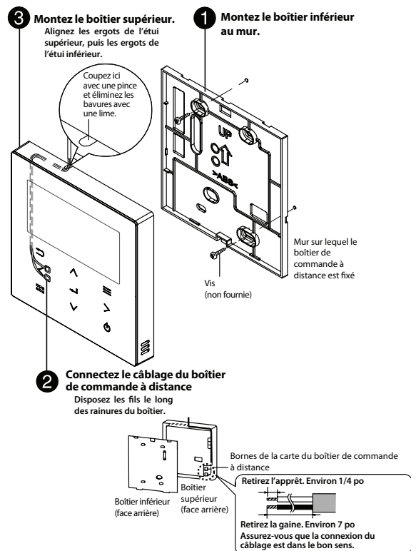
Figure 6-12 Instructions de montage - en surface
