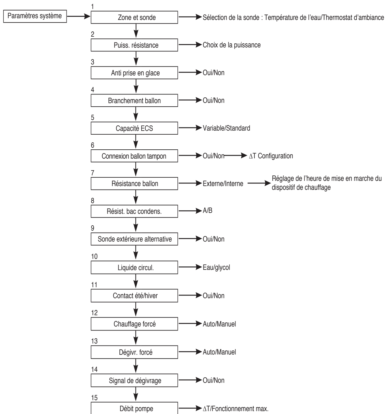
Figure 6-25 Organigramme du boîtier de commande à distance
