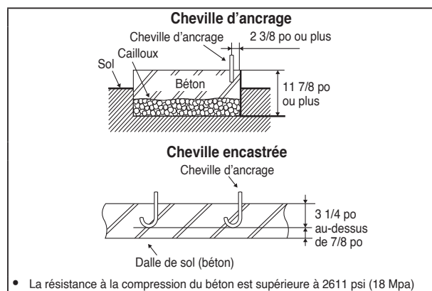
Figure 6-1 Cheville d'ancrage contre cheville encastrée
