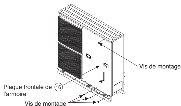
Figure 6-6 Retrait de la plaque frontale de l'armoire
