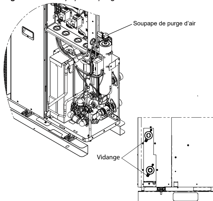
Figure 6-16 Soupape de purge d'air
