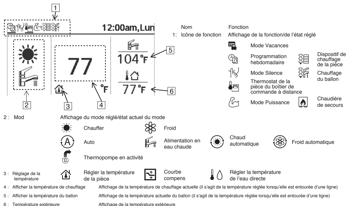
Figure 6-23 Écran d'accueil du boîtier de commande à distance
