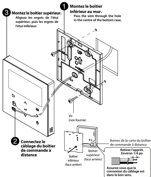
Figure 6-13 Instructions de montage - encastré
