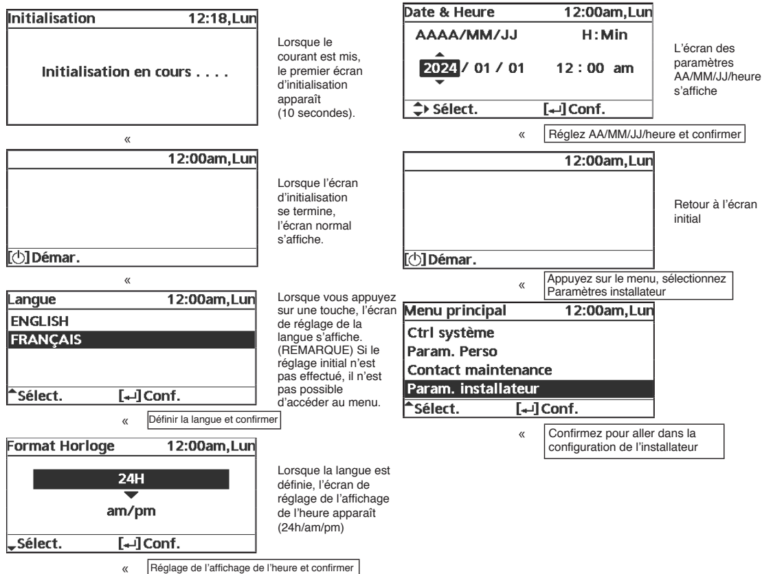
Figure 6-24 Initialisation du boîtier de commande à distance
