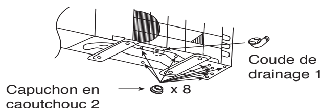
Figure 6-2 Vidange de l'unité
