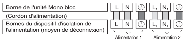
Figure 6-8 Exigences en matière de dénudage et de connexion des câbles
