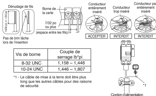
Figure 6-8 Exigences en matière de dénudage et de connexion des câbles
